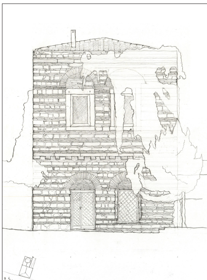
5. kép. Az erdélyi követek házának délkeleti homlokzatáról készült helyszíni, kézi manuálé (Készítette: Kulcsár-Kilyén Róbert, 2019)
