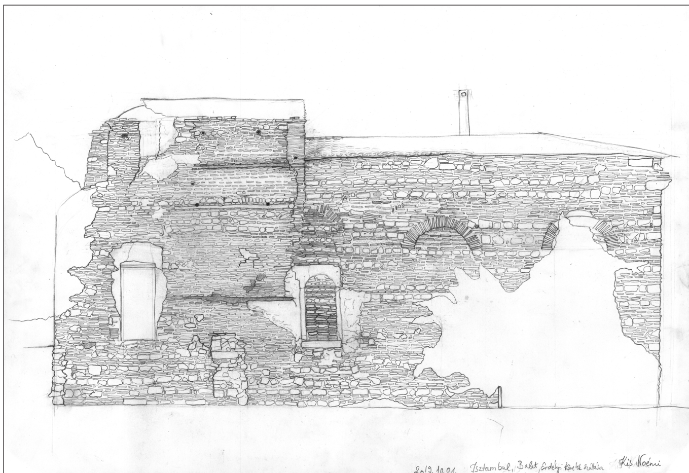
3. kép. Az erdélyi követek házának délnyugati homlokzatáról készült helyszíni, kézi manuálé (Készítette: Kis Noémi, 2019)
