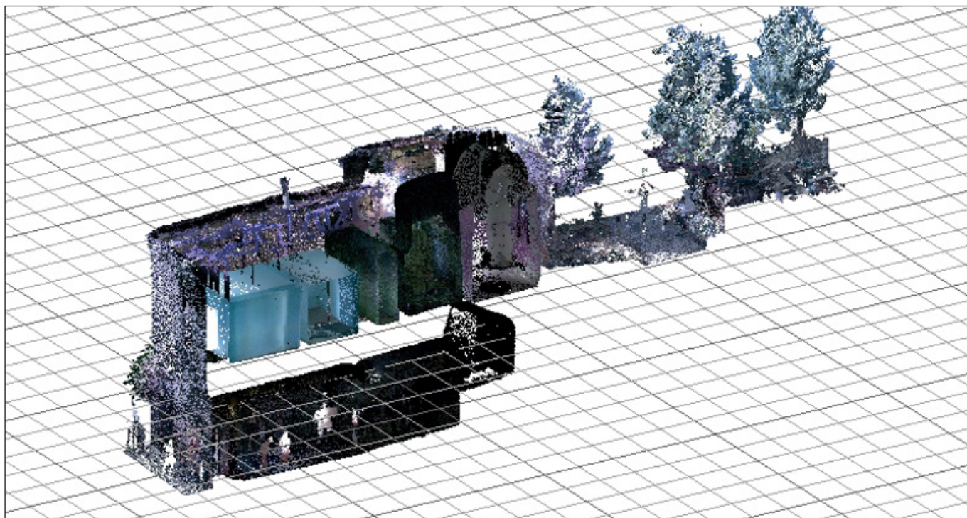
7. kép. Az erdélyi követek házáról készült pontfelhő-metszet (Készítette: Kovács Máté Gergő, 2019)
