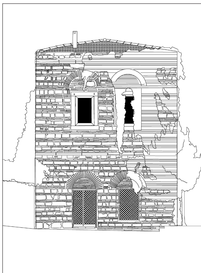
6. kép. Az erdélyi követek házának délkeleti homlokzatáról készült digitális felmérési rajz (Készítette: Kulcsár-Kilyén Róbert, 2019)
