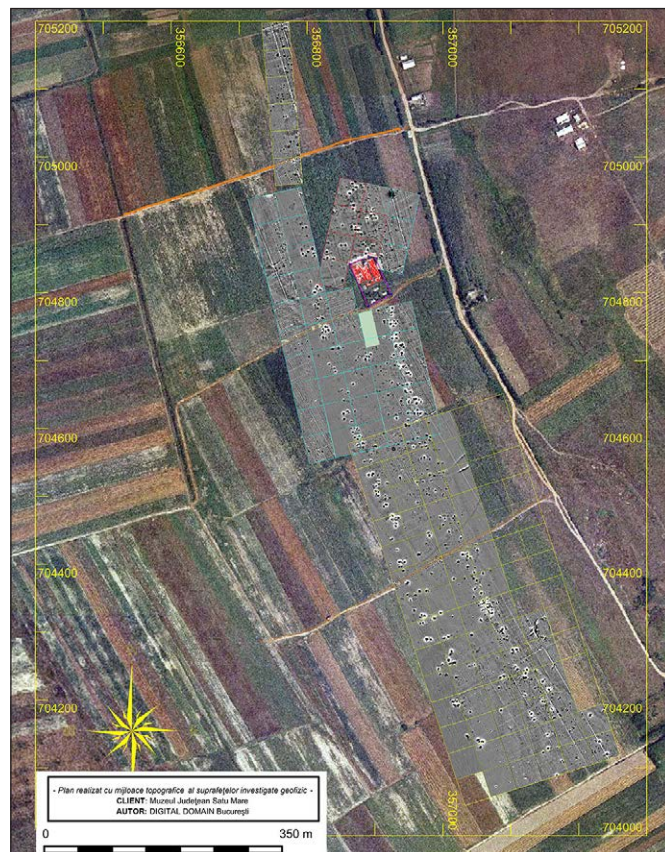
9. kép: Geomágneses felmérés az aranyosmeggyesi (Medieșu Aurit) fazekastelepen. A fehér „árnyékkal” körülvett fekete pontok edényégető kemencéket jeleznek. Megfigyelhető, hogy ezek két sávban helyezkednek el, közöttük utcaszerű térrel. Keleti irányban a lelőhelyet a Racta patak ártere határolja, és nyugati irányban is egy lapályos területtel határos. Dél és észak felé a lelőhely kiterjedését még nem sikerült megállapítani.
