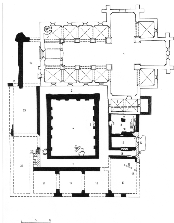
► 3. kép. A bélapátfalvi ciszterci kolostor alaprajza (Valter Ilona, „Kisebbségi régészeti kutatás a bélapátfalvi volt ciszterci apátság temploma mellett,” Műemlékvédelem 49 (2005): 339.)
