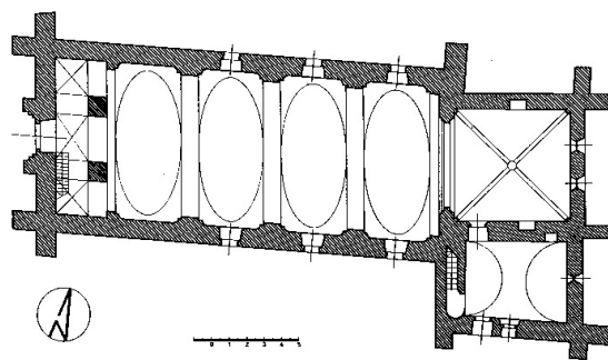
► 6. kép. A mórachidai premontrei prépostsági templom alaprajza (Valter Ilona, Romanische Sakralbauten Westpannoniens (Eisenstadt: Roetzer, 1985), 74.)
