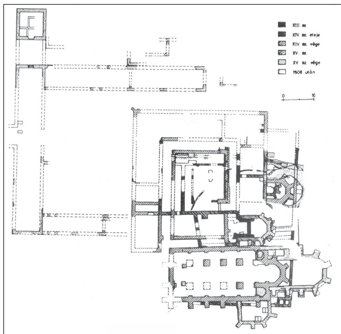
9. kép. A budaszentlőrinci kolostor alaprajza (BENCZE–SZEKÉR 1993, 38)
