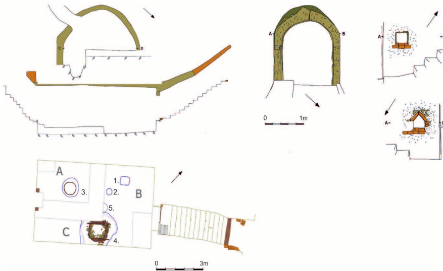
2. kép: A pince alaprajza és metszetei a feltárás után, valamint a teherlejáró kőkerete és a lépcső aljában kétoldalt téglából kialakított mécsstartók
