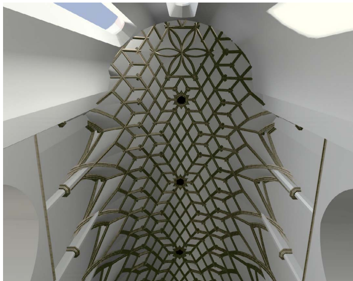
6. kép: A szentély boltozatának rekonstrukciója
