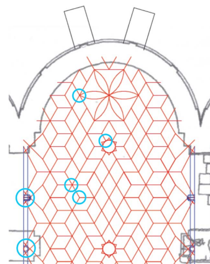
4. kép: A templom szentélyének boltozatrekonstrukciója a fennmaradt bordacsomópontok helyének jelzésével
